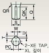
축단상세도
