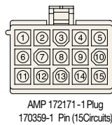
Incremental 엔코더 Connector 접속도
