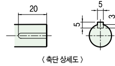
(측단 상세도)
